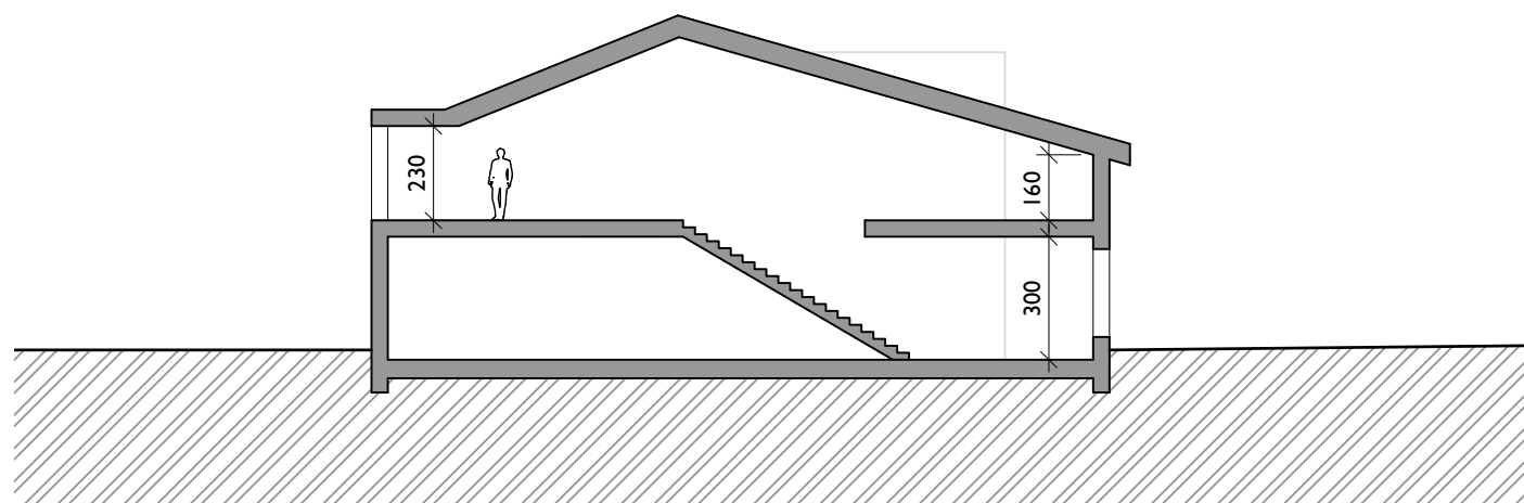
Coupe AA
